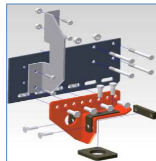
Tažná koule ( Z 75 ) Konzola taž. zařízení ( Z 75 ) Spec. mont. konzoly ( Z 75 )
